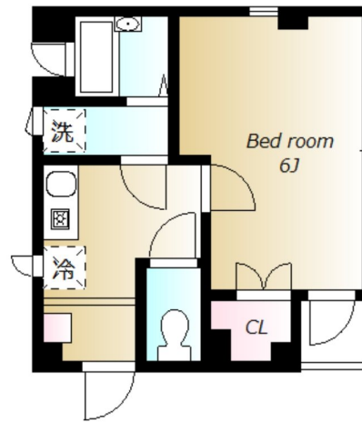
【間取り図】
