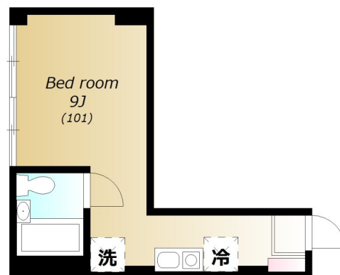
【間取り図】
